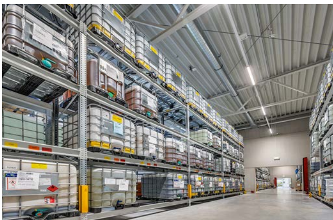
Im Gefahrgutlager bieten die Galler Omega-Palettenregale Platz für 204 IBC-Container.
